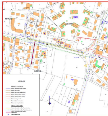
Renouvellement en Ø 160 mm FONTE sur 230 ml Estimation SOCAMA : 120 000,00 € HT
